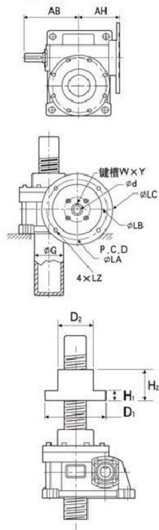
GLFSJD型尺寸
