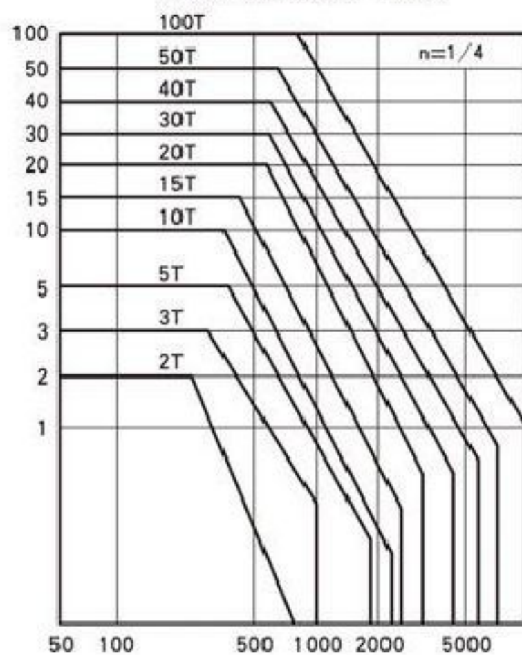
许用弯曲负荷 (吨)
