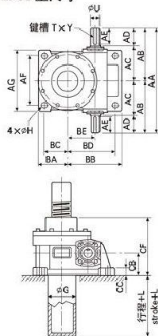
GLFSJ型尺寸
